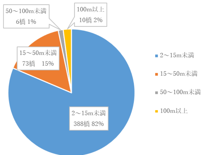
図-2 橋長別の橋梁数分布
