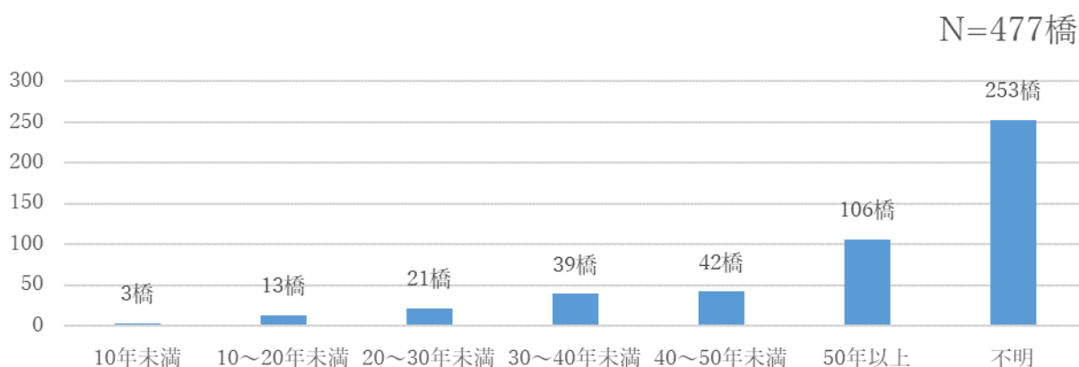
図-3 供用年数別の橋梁数分布
