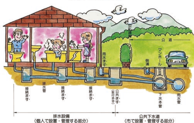
排水設備の設置例 (分流式公共下水道の場合)
