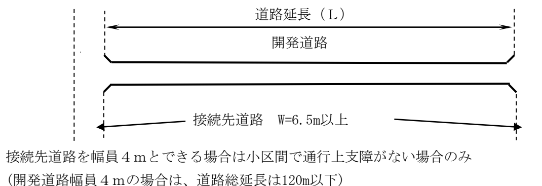
図 3-5 通り抜け道路
