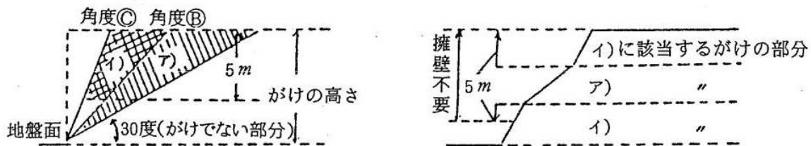
図3-9 擁壁を要しないがけ又はがけの部分 図3-10
