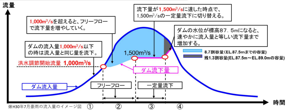
【洪水調節図】
