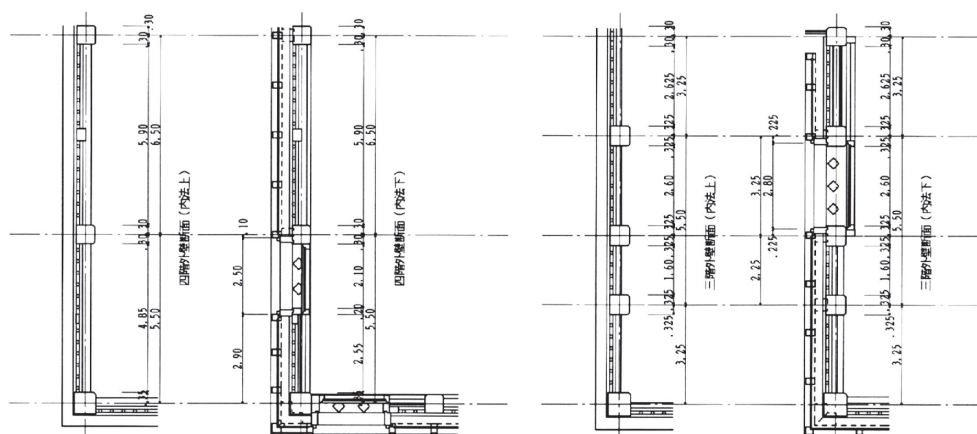
梁行矩計詳細図-2 (天守3, 4階)
