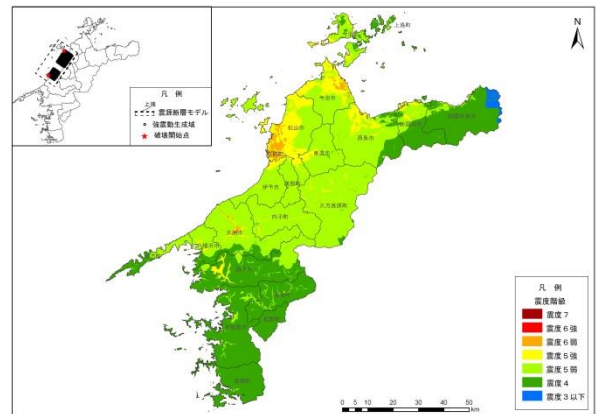
②安芸灘～伊予灘～豊後水道のプレート内の地震（北側）の震度分布 (2 ケースの重ね合わせ)
