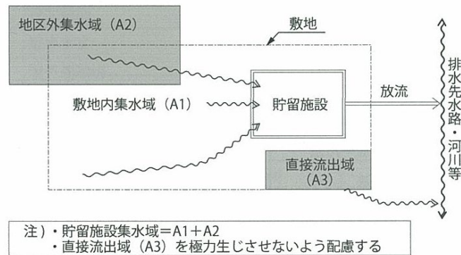
図-10 貯留施設と集水域等の調査
