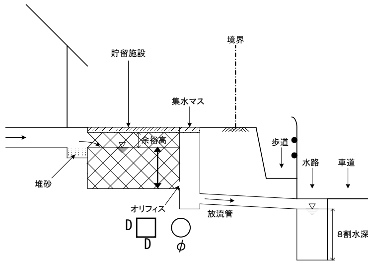
図-18 放流施設の計画
