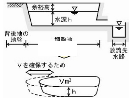
図-17 貯留施設形状の計画
