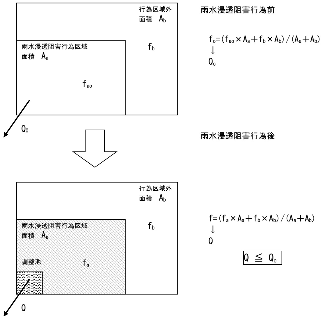
図-24 集水域模式図
