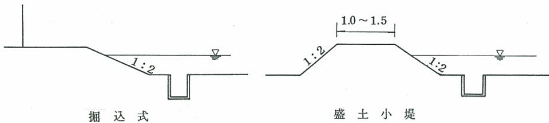
図-20 貯留部周囲堤の概念
