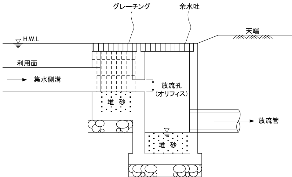
図-16 放流施設構造図
