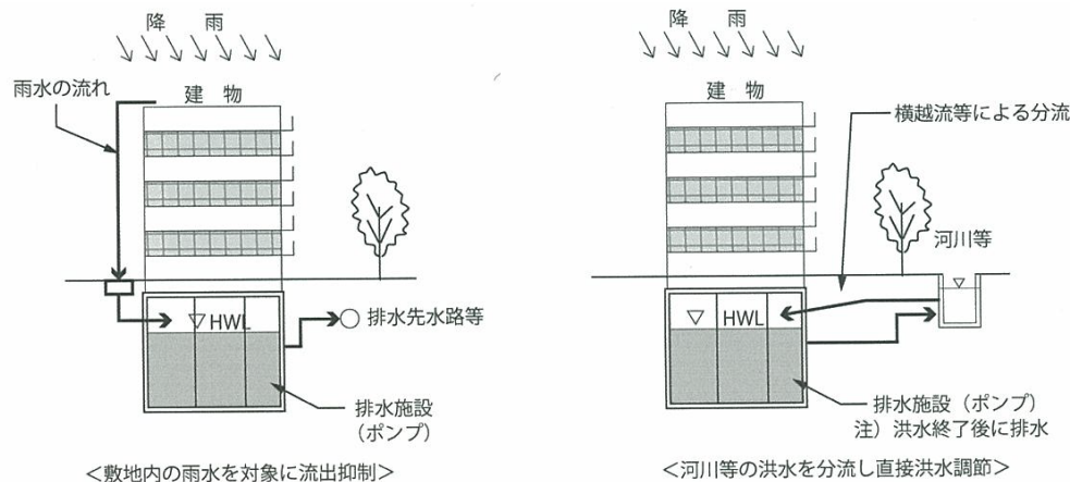
図-13 雨水の流入方式の概念
