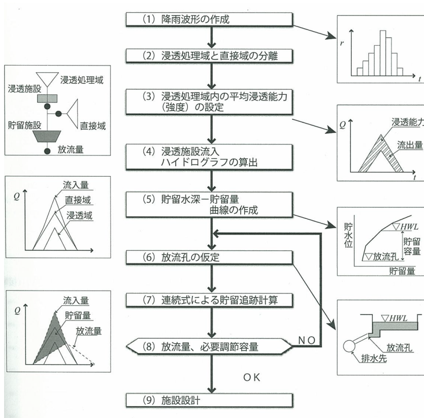
図-15 貯留施設と浸透施設併用における流出抑制手法の概念
