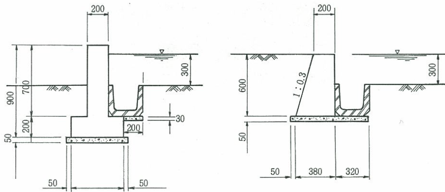
図-21 周囲小堤としてのコンクリート壁の構造例
