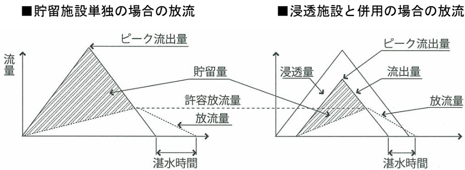
図-14 浸透施設による湛水時間短縮の効果（概念）
