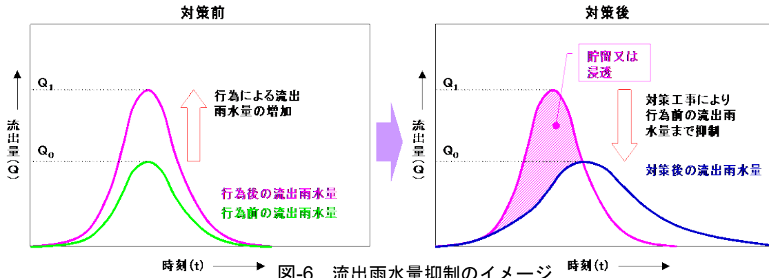
図-6 流出雨水量抑制のイメージ
