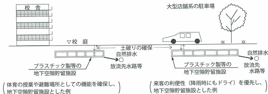
図-12 地下空隙貯留施設の概念
