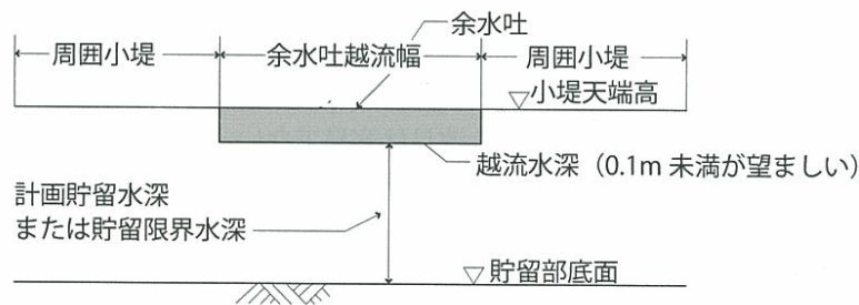
図-22 余水吐と小堤天端高
