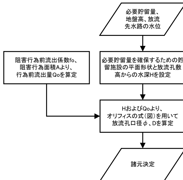
図-19 放流施設の設計フロー
