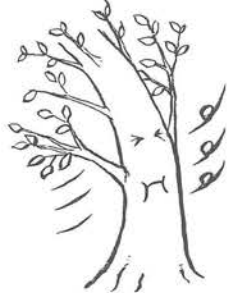
木は風の力等をまともに受けないように、しなったりして力を受け流します。しなるとき木の表面は、力の影響を一番受けます。逆に木の中心部分は、それほど力を受けません。木に空洞ができても幹の中心がなくなっても倒れないのはそのためです。
