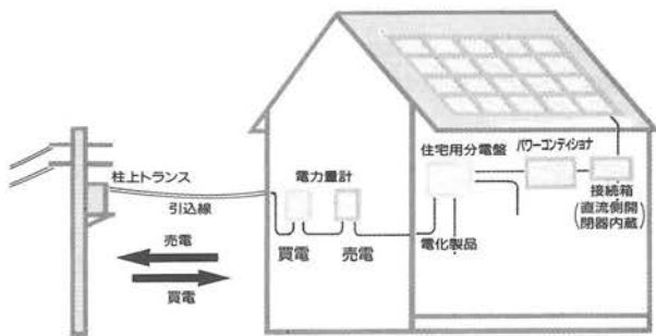
太陽光発電システムイメージ図
