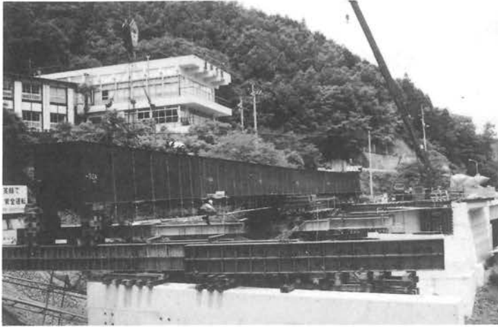
150トンのトラッククレーンを使い桁を移動
