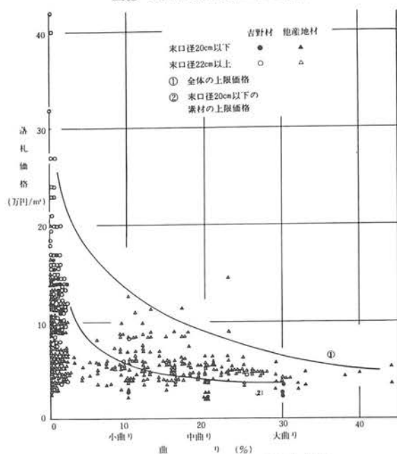
図3 スギにおける素材の曲りと材価
