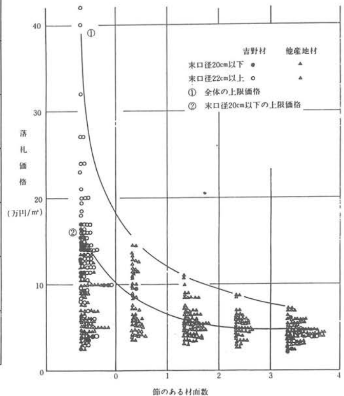
図4 スギにおける節のある材面数と材価
