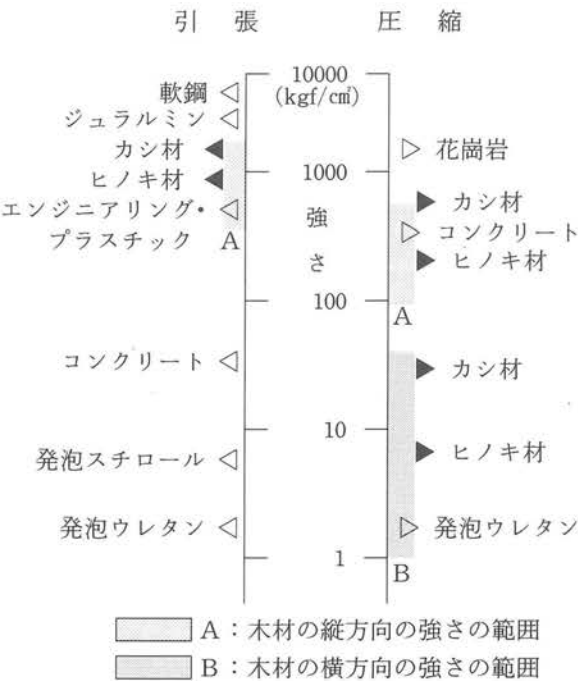
図1 種々の材料の強さの比較
