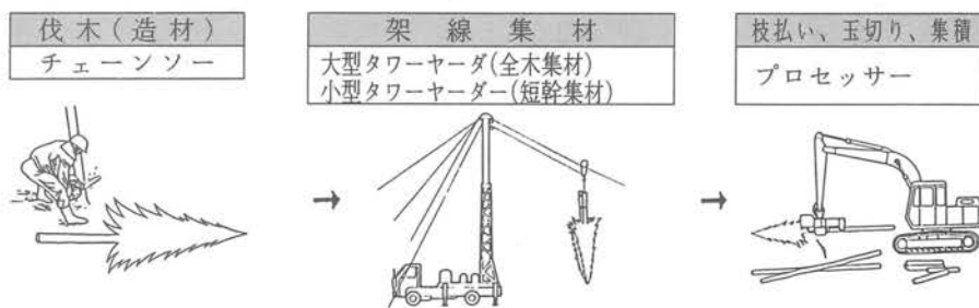
図-2 タワーヤーダー
