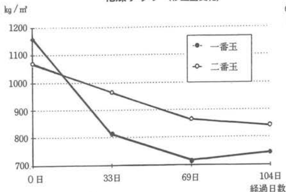
乾燥グラフ (杉重量変化)
