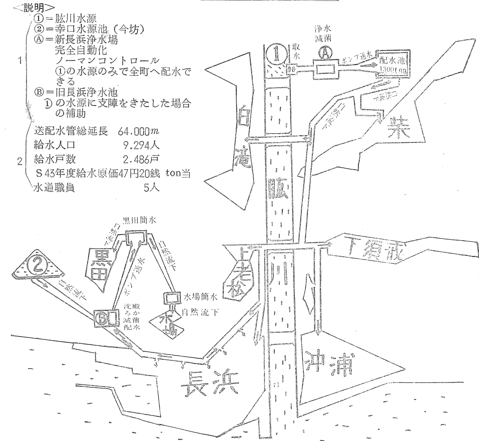
長浜上水道配管図
