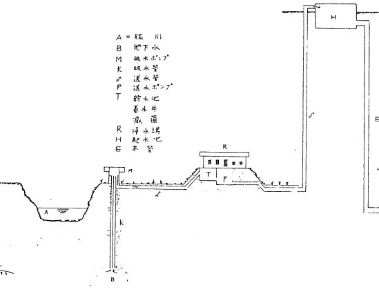
長浜水道浄水場略図
