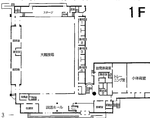
総合体育館平面図
