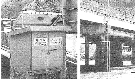
潮位に連動した河川水位と塩分濃度の調査状況
