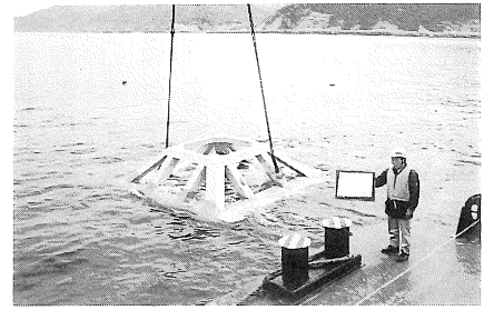
良好な漁場造成を図る魚礁設置状況
