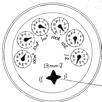
円読式水道メーター
