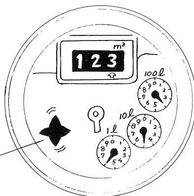
直読式水道メーター
