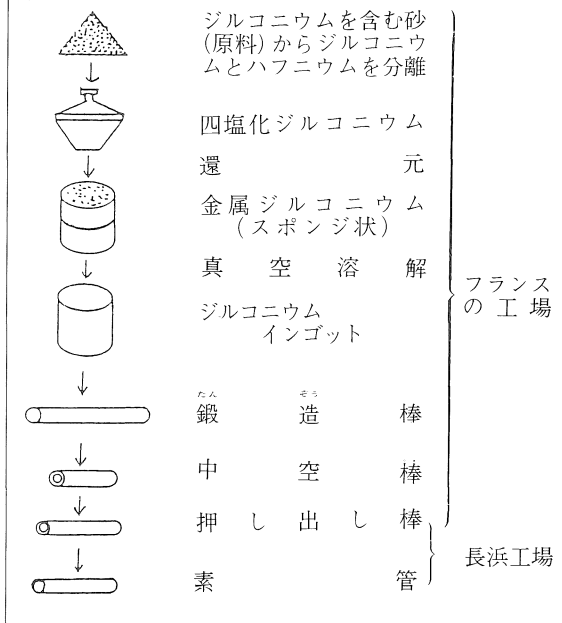
(図1) ジルコニウムから製品までの製造工程
