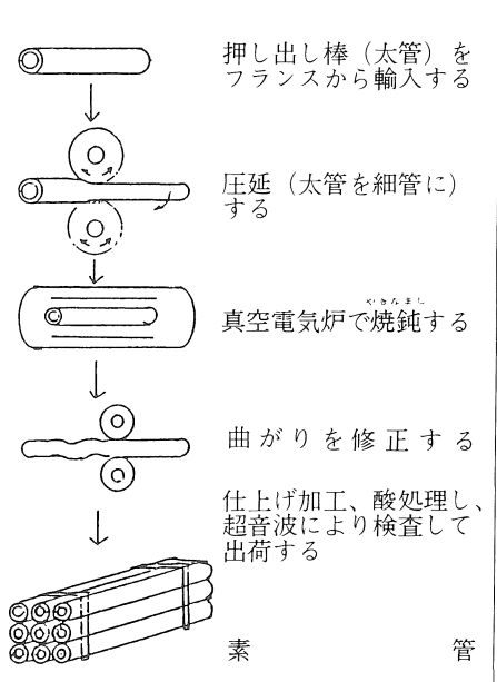
(図2) 長浜工場の製造工程
