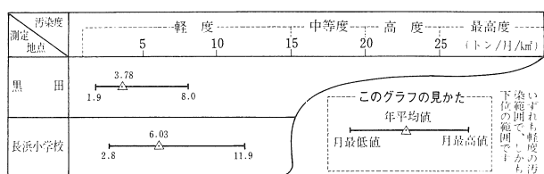
デボジットゲージ法による降下ばいじんの測定結果(48年度分)
