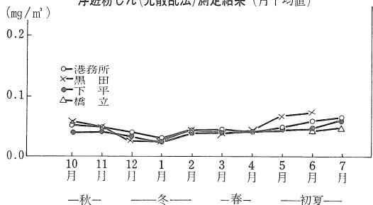
浮遊粉じん(光散乱法)測定結果(月平均値)
