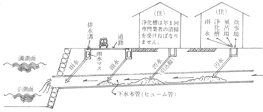
下水道のしくみ（合流式）
