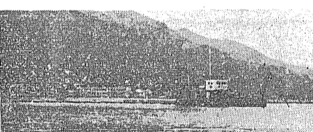
【写真説明】 (左上) 砂利を送る鉄管(長浜大橋から撮影) (右上) 1日に約400m³の砂利を吐き出します (右) 舷川河口の州の砂利を送るサンドポンプ。
