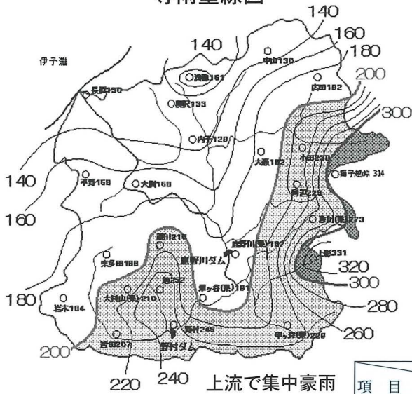
等雨量線図
