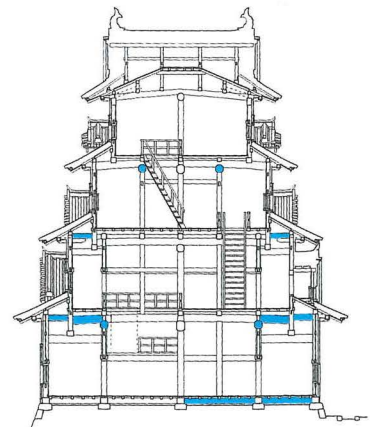
▲図1 天守桁行断面図 着色した部分に部材を追加している
