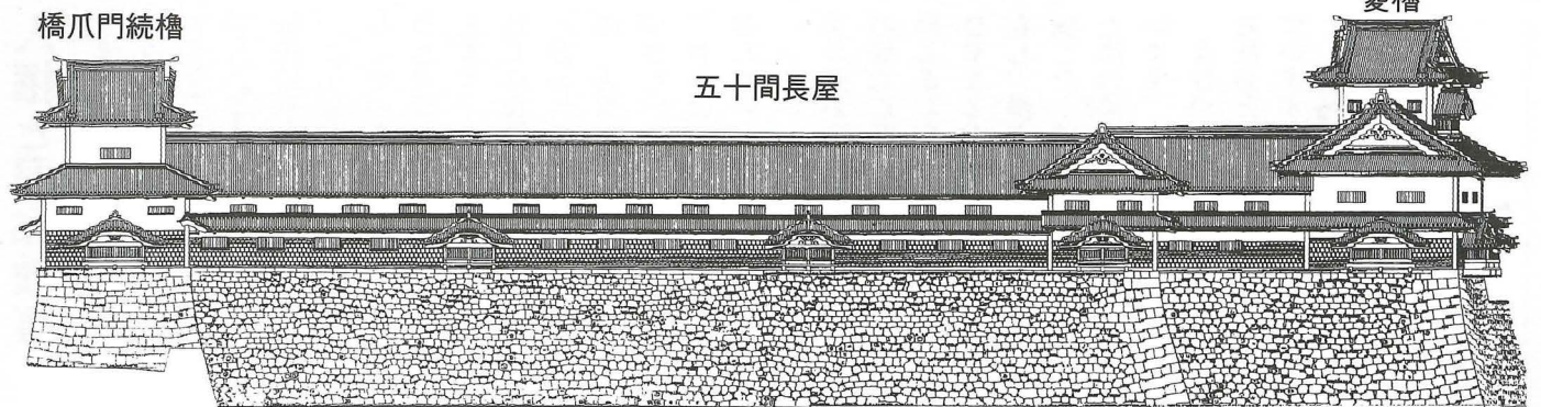
▲復元立面図
