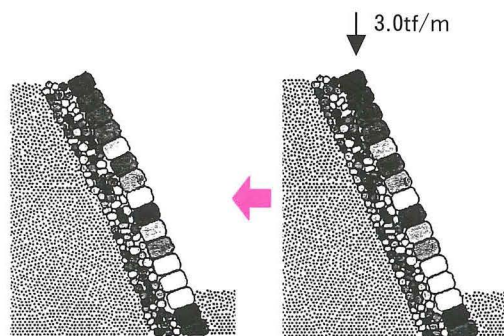
天守台石垣に天守閣壁の荷重がかかる場合(250ガル)
