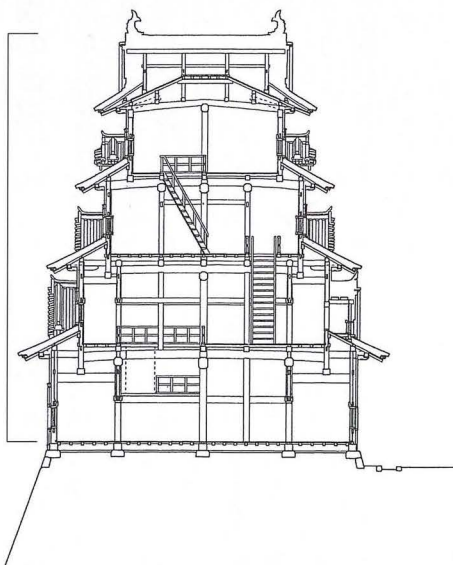
▲図2 天守桁行断面図(実施設計)
