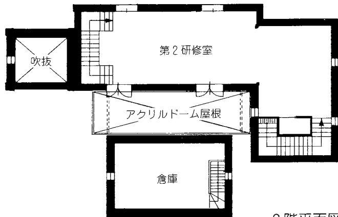
2階平面図
