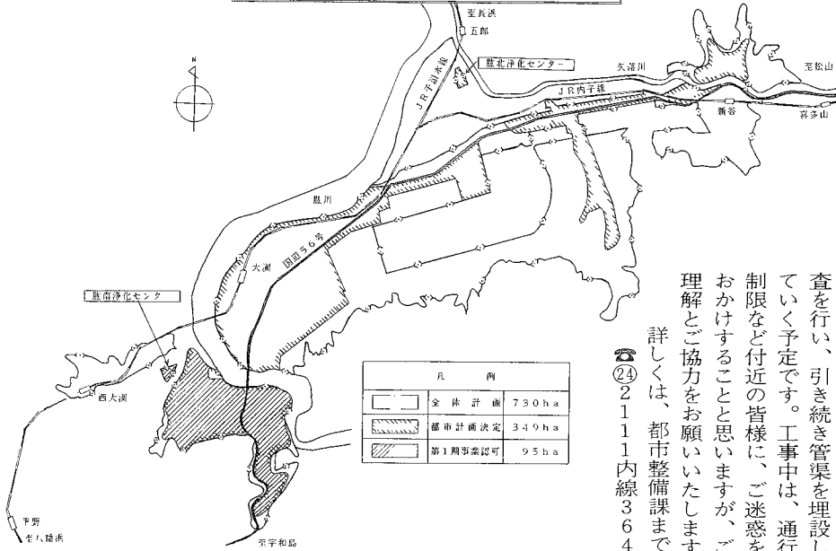
公共下水道一般平面図
