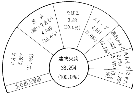
建物火災の主な出火原因(S 59年度)
