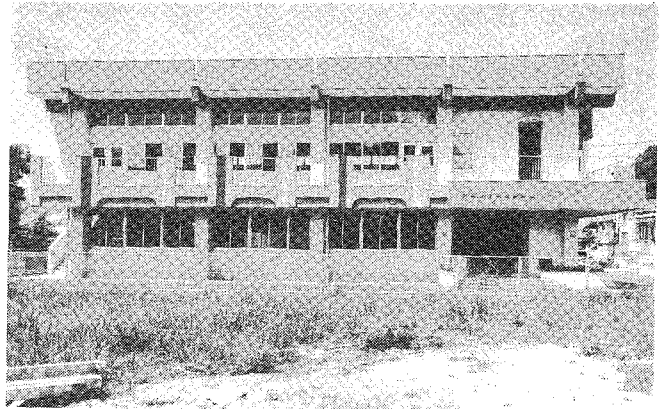
大洲隣保館 鉄筋コンクリート造2階建、598平方メートルの近代的な建物で、学習、集会など幅広い用途に利用できるようになっています。
